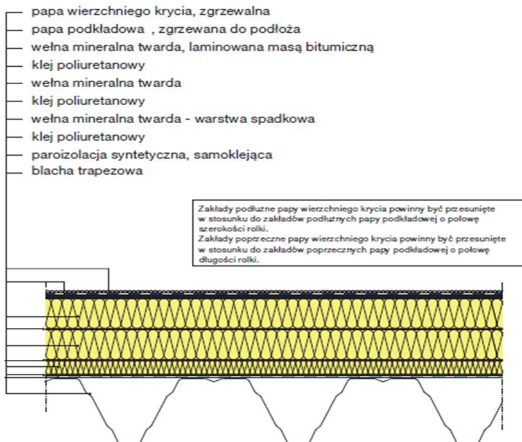
Rysunek poglądowy ułożenie warstw pokrycia dachowego
